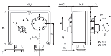
BITERMOSTATO AD IMMERSIONE 623000
