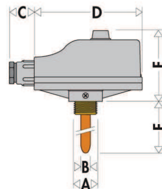
TERMOSTATO AD IMMERSIONE A RIARMO 624000
