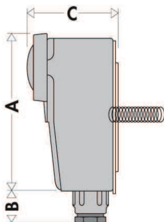
TERMOSTATO A CONTATTO 621000
